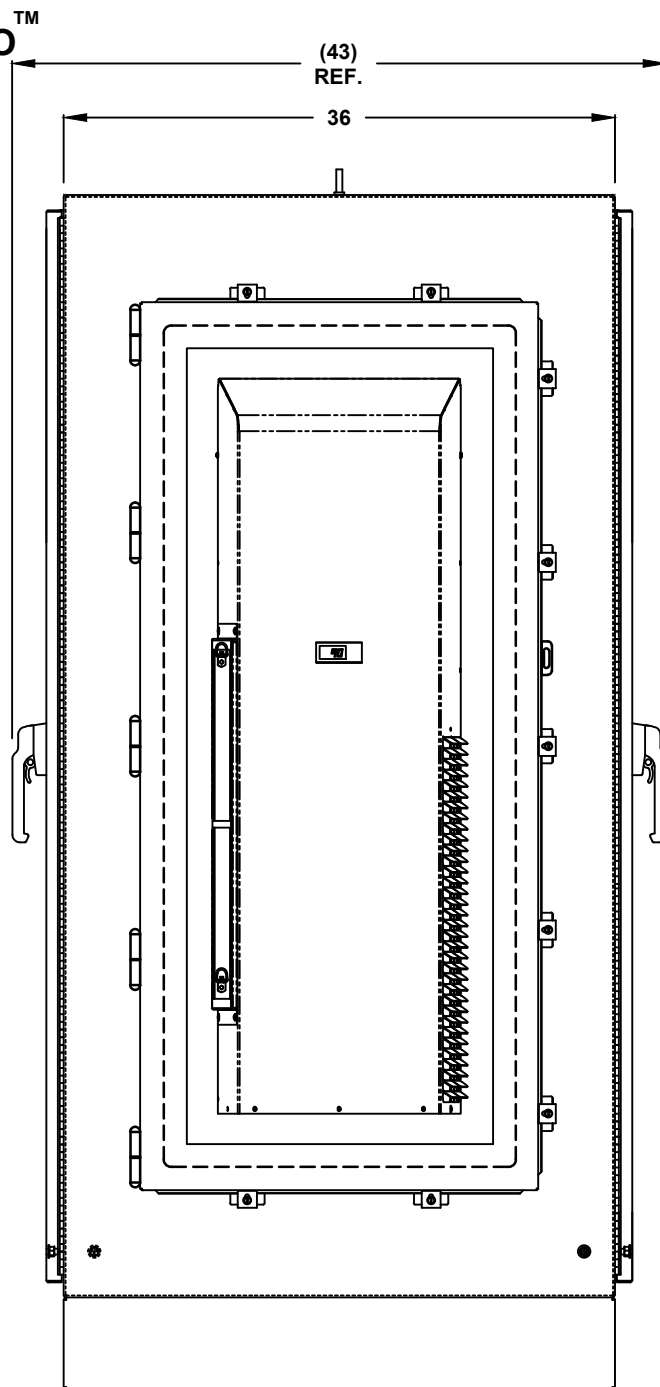
LEFT SIDE
